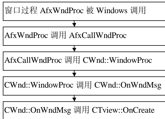
图 4-2 标准 Windows 消息的处理。下面描述每一步的详细处理。
