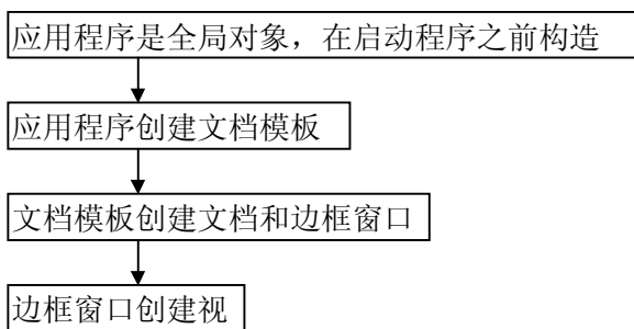
图 5-1 应用程序创建 MFC 对象的顺序
