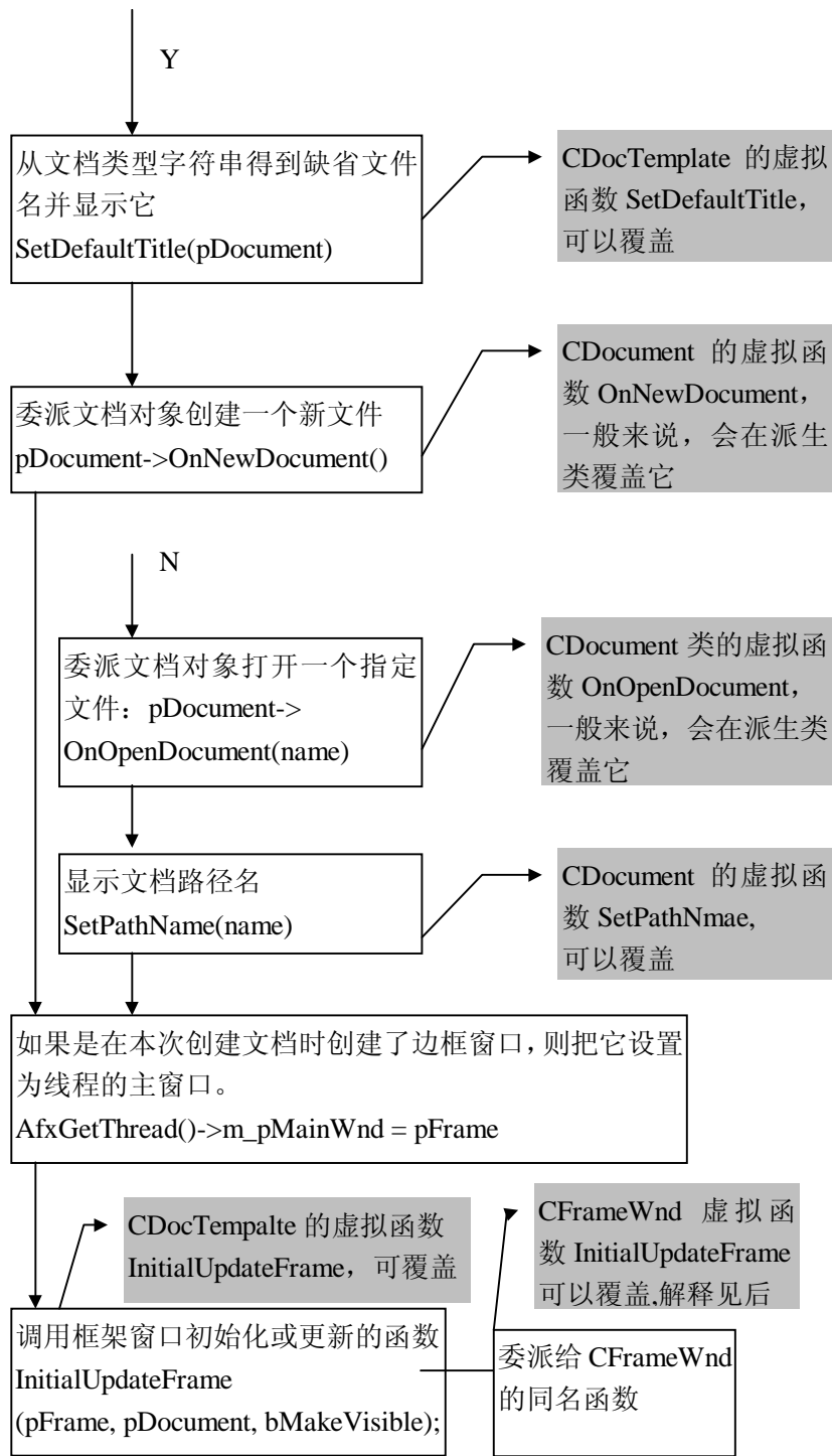
图 5-8 CSingleDocTemplate 的 OpenDocumentFile 函数
