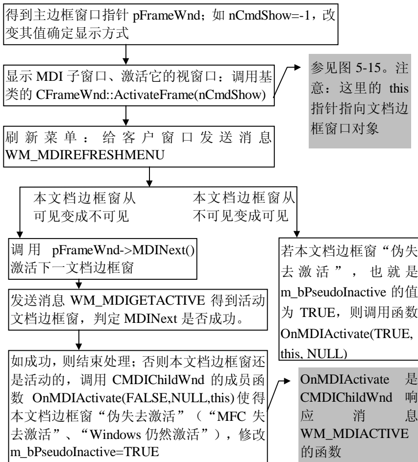
图 5-18 CMDIChildWnd 的 OnActiveFrame 函数
