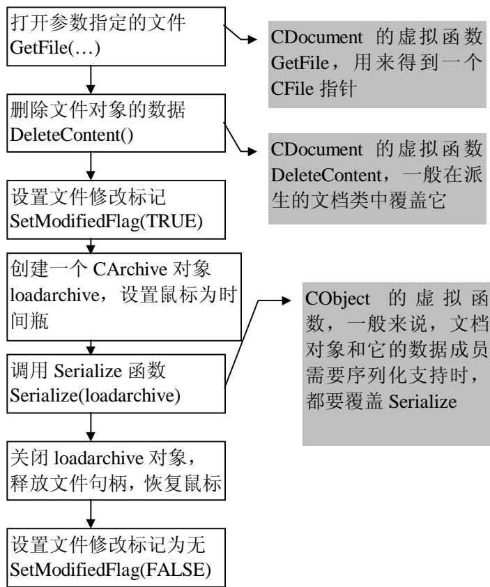
图 5-10 CDocument 的 OpenDocument 函数
