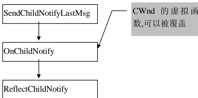
图 4-4 消息反射的处理流程
