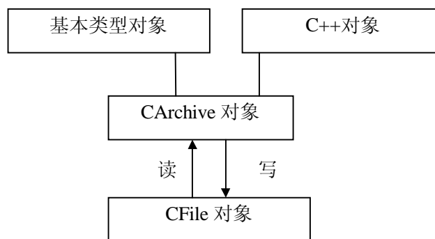
图 3-2 序列化的机制
