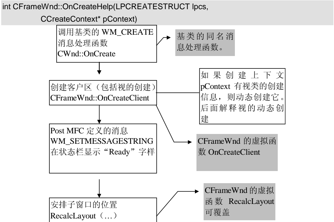
图 5-12 CFrameWnd 的 OnCreateHelp 函
